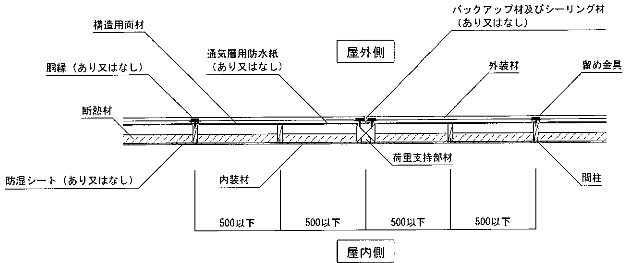
水平断面図
